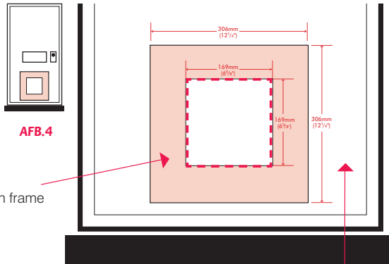
PVC/uPVC/metalen deur
